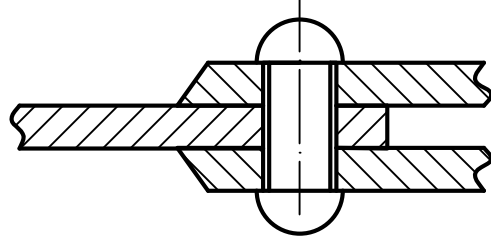
Çift Bindirmeli Perçinleme
