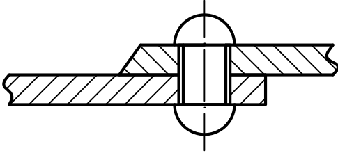
Tek Bindirmeli Perçinleme
