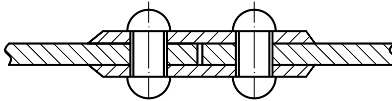
Çift Yamalı Perçinleme
