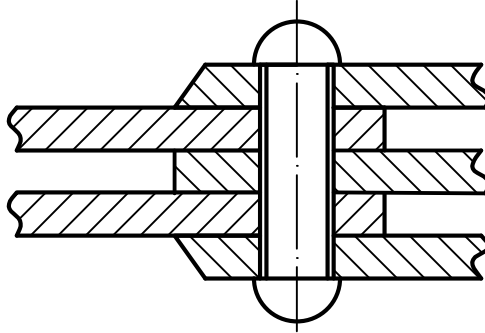
Çoklu Bindirmeli Perçinleme
