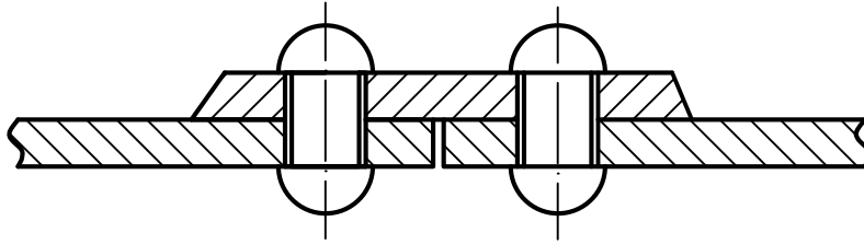
Tek Yamalı Perçinleme
